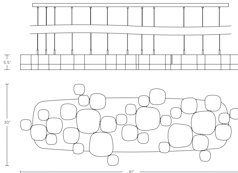
MULTI-MODULE CHANDELIER, 5 + 7 + 11 + 11
